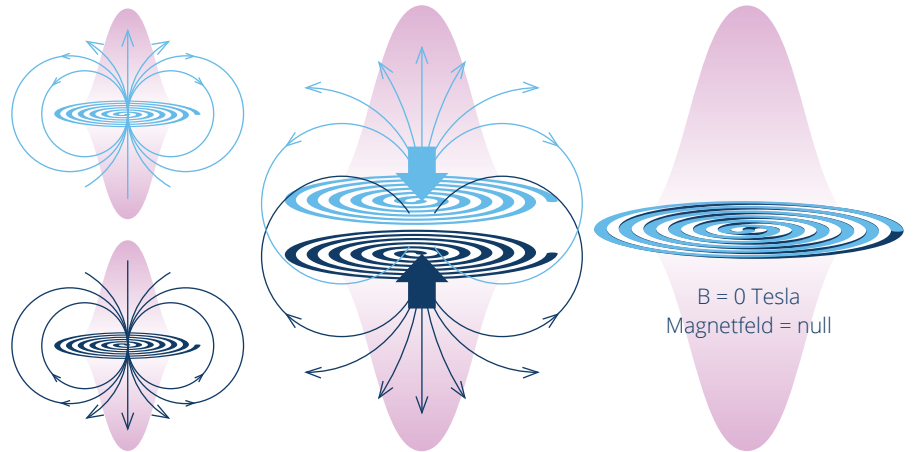
■ ■ Magnetfelder ■ Quanten-Potential (Vektorpotential)
